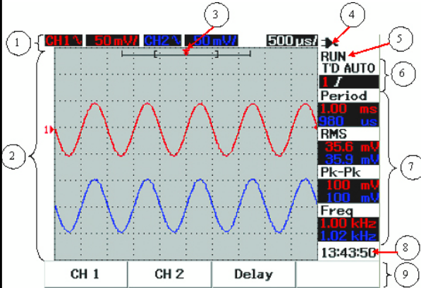
Figura 1 Pantalla del Osciloscopio
